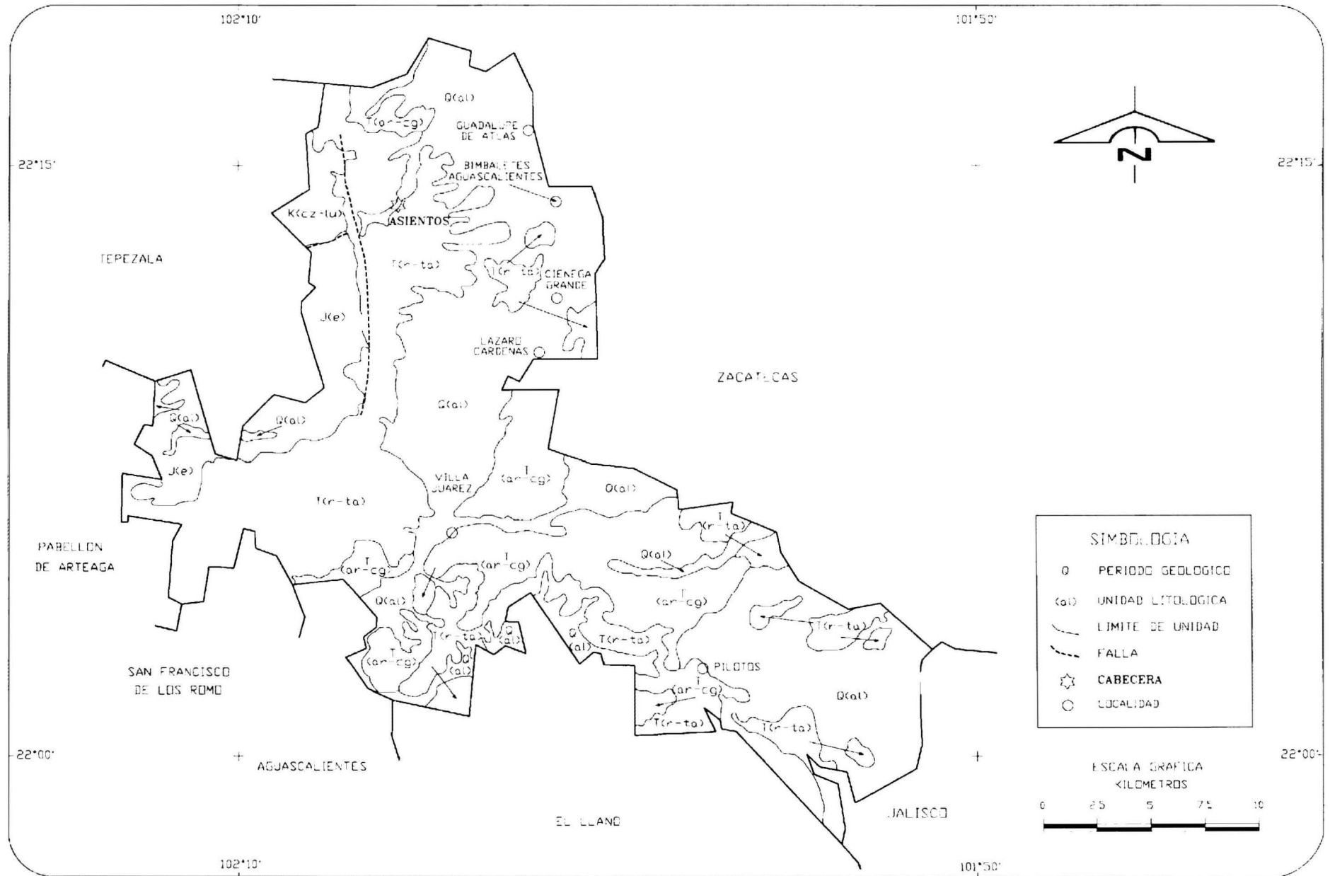
FUENTE: CGSNEGI. Carta Geológica, 1:250 000.
